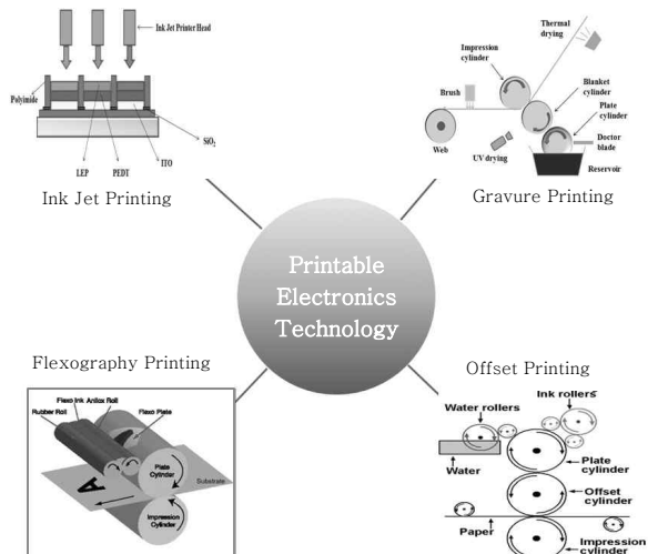
그림 2 Schematic of printable electronics printing process 17,28)
