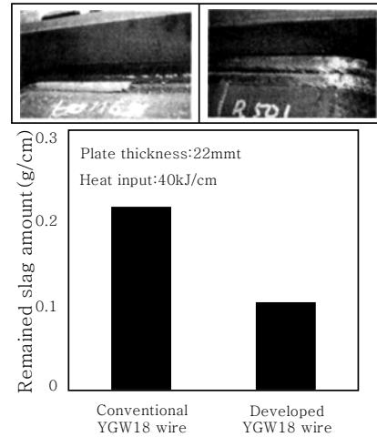
그림 2 로봇용접용 YGW18 Solid wire의 Slag발생량 비교
