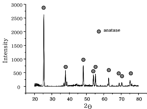
Fig. 1 XRD data of pure TiO 2 powder
