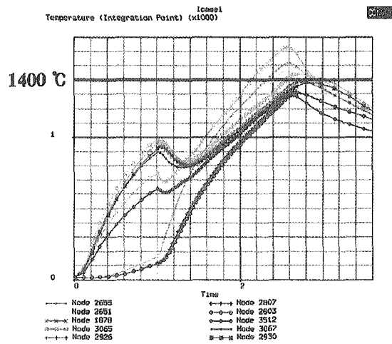
(b) Thermal cycle
