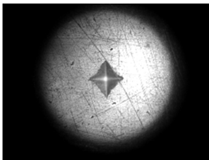
Fig. 3 Indentation mark (Hv)
