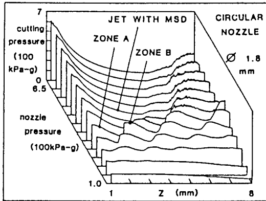
그림 5. 절단압력 12)
