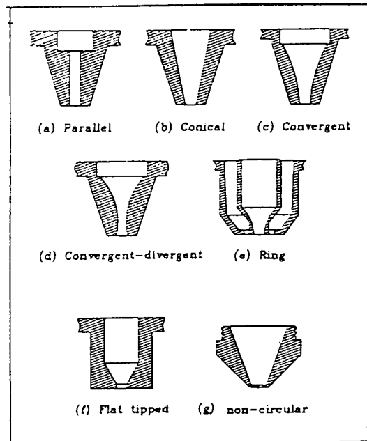
그림 8. 일반적인 노즐 12)
